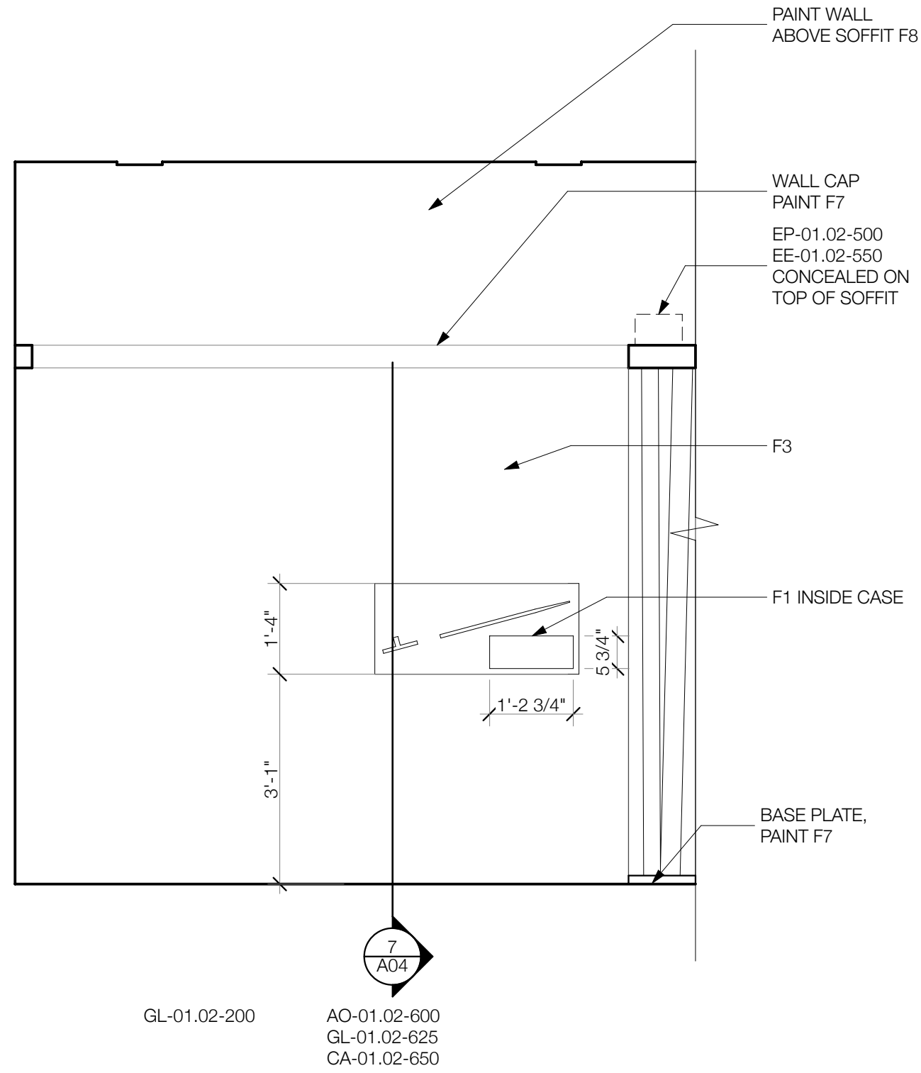
PIPE DISPLAY ELEVATION
