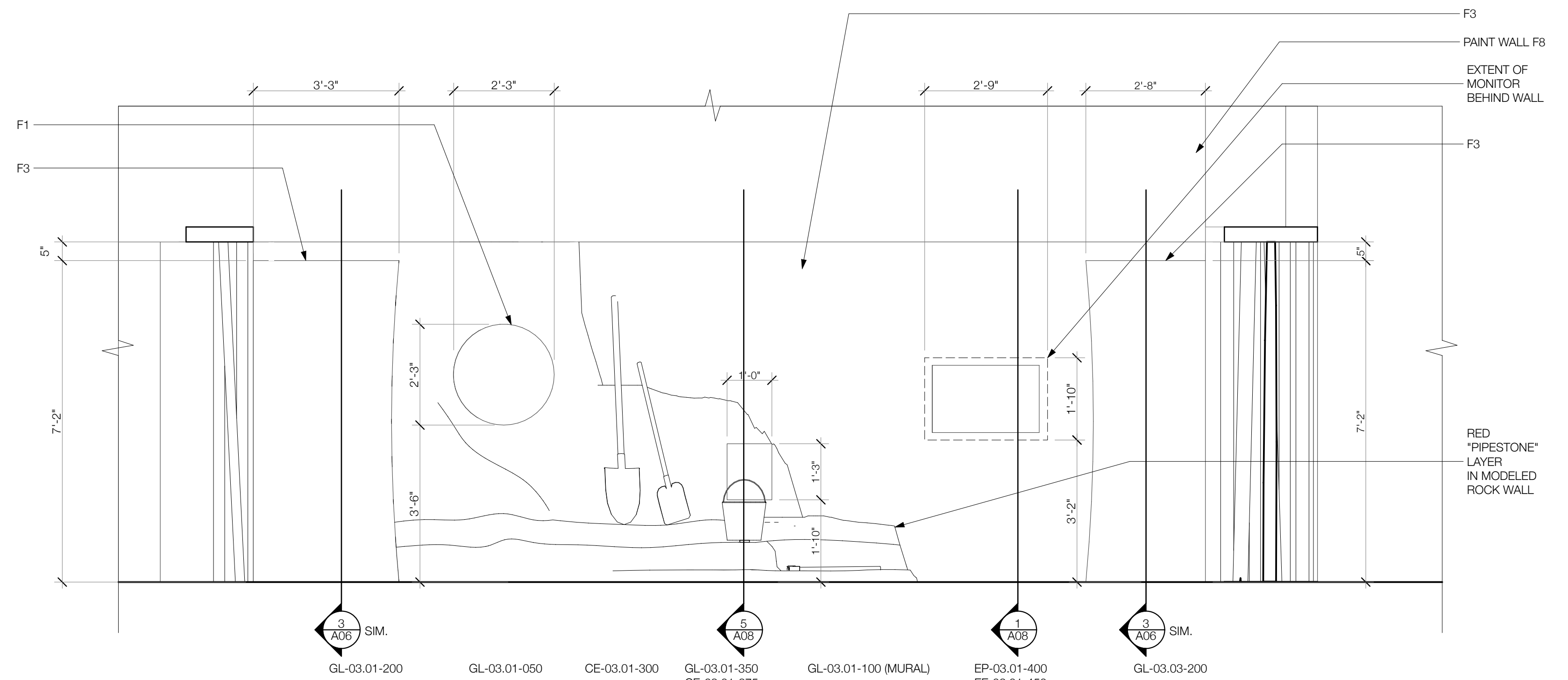
ROCK WALL ELEVATION SCALE: 1/2" = 1'-0"
